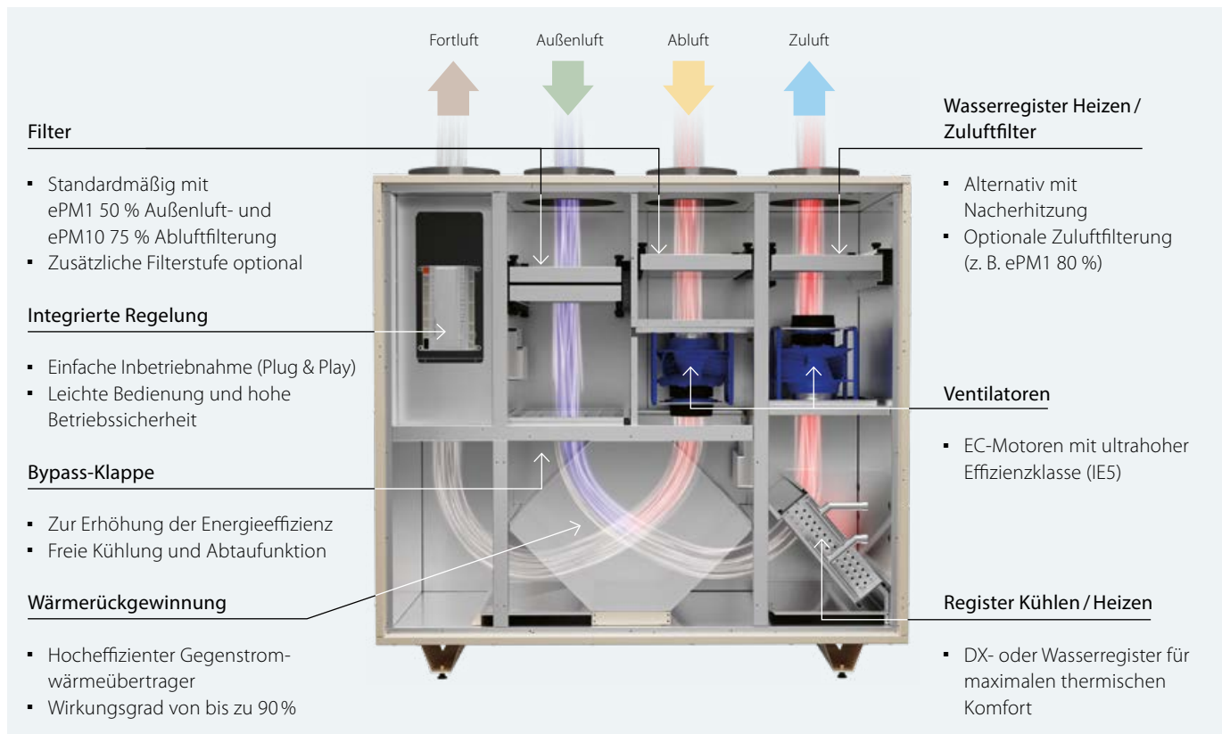
Abb.: Winterbetrieb; Modell mit Bedienseite rechts. Das Modell mit Bedienseite links ist spiegelsymmetrisch aufgebaut.
