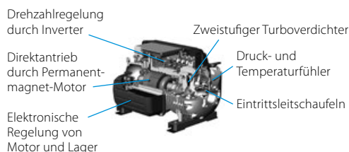
Innovativer Turboverdichter mit Magnetlagern
