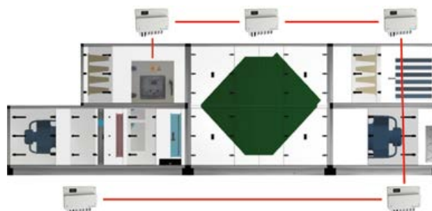
Dezentrale Steuerplatine des digitalen Regelungskonzeptes
